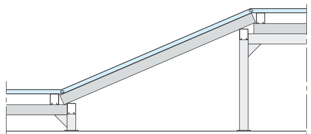
Variante con perfilera ligera de acero
