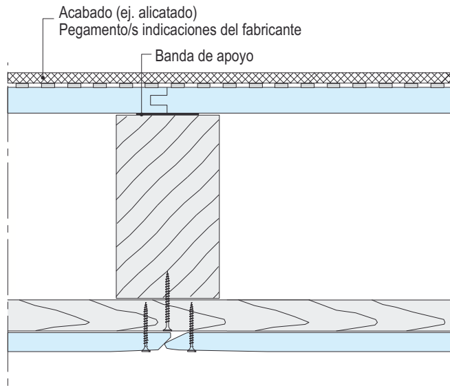
F191-V9 Apoyo sobre viga de madera
