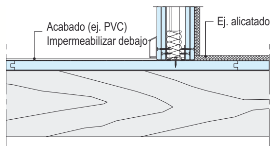
F191-V11 Tecnofloor V sobre vigas y sistemas Knauf W112 (Esc. 1:10)
