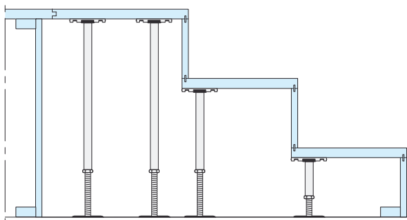
Sección vertical: con pedestales
