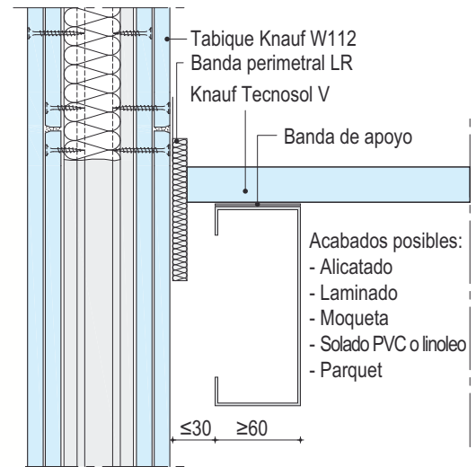
F191-V1 Acabado sobre perfil ligero y encuentro con tabique Knauf W112
