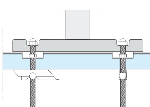
Mesa de director de orquesta anclada directamente a la placa de suelo con taco Fischer KD 8
