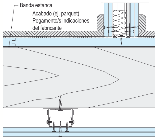
F191-V12 Tecnofloor V con solado de parquet y sistemas Knauf W112 y D112
