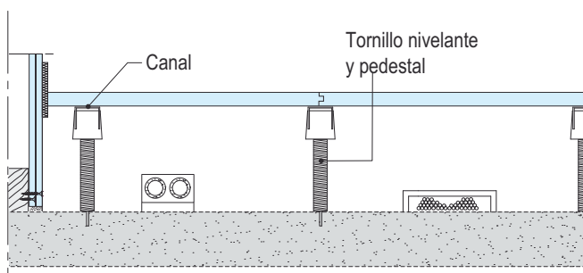
F191-V18 Tecnosol V sobre apoyos Sistema Granab 7000 (Esc. 1:12,5)
