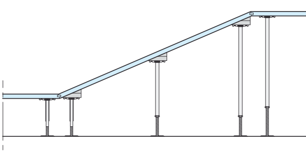
Variante con pedestales y cuñas
