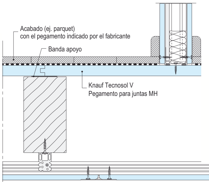
F191-V15 Tecnosol V con solado de parquet y sistemas Knauf W112 y D112
