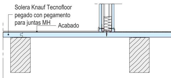
F191-V14 Tecnofloor V sobre vigas de madera y sistemas Knauf W111 (Esc. 1:10)
