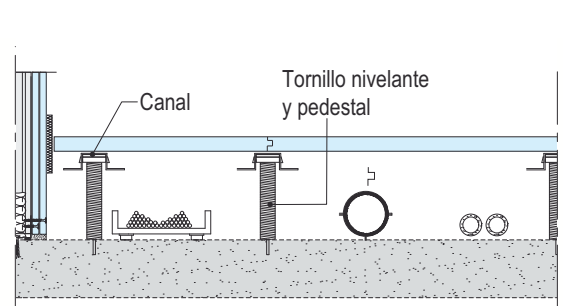
F191-V17 Tecnosol V sobre apoyos Sistema Granab 100 (Esc. 1:12,5)
