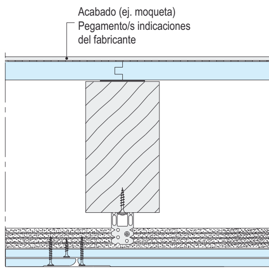
F191-V7 Tecnofloor V conjunto con Techo Knauf D112
