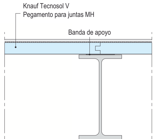
F191-V5 Tecnosol V sobre perfiles estructurales
